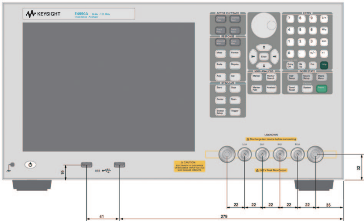
图 10. 前视图 (毫米)
