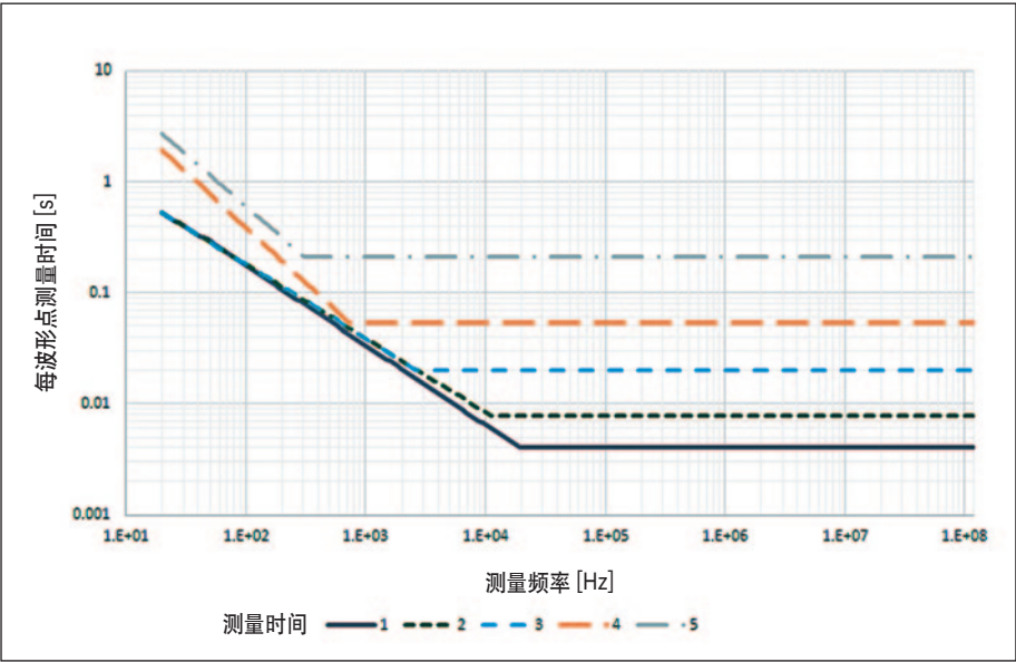
图3. 测量时间(选件120, 适配器: 7毫米42942A/ 探头42941A, 典型值)
