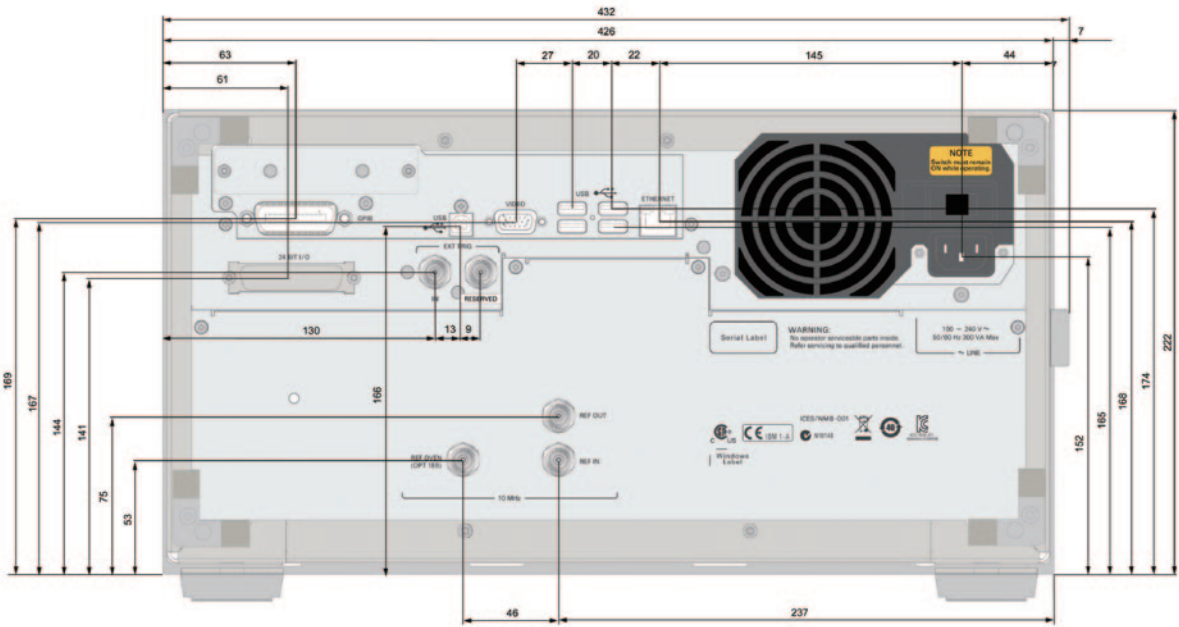
图 11. 后视图 (毫米)
